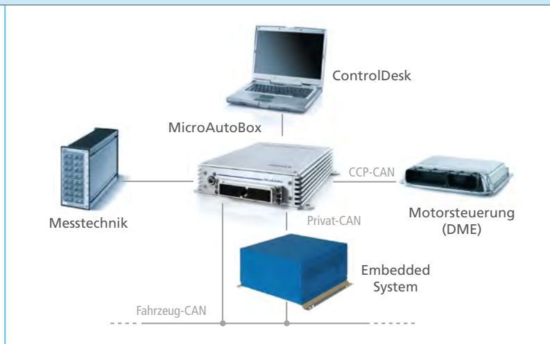
Abbildung 3: Hardware- und Kommunikationsstruktur im Versuchsträger.
